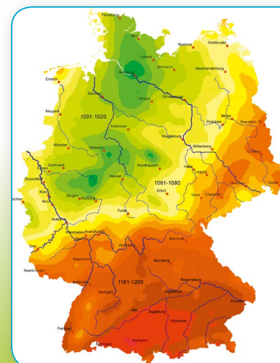
Globalstrahlung in Deutschland 2012 Quelle: Deutscher Wetterdienst
